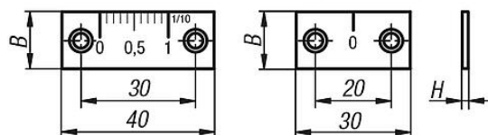
Nonio Linea dello zero
