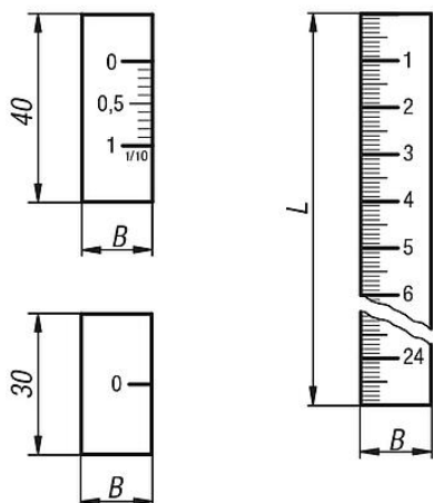
Autoadesivo Posizione di montaggio verticale
